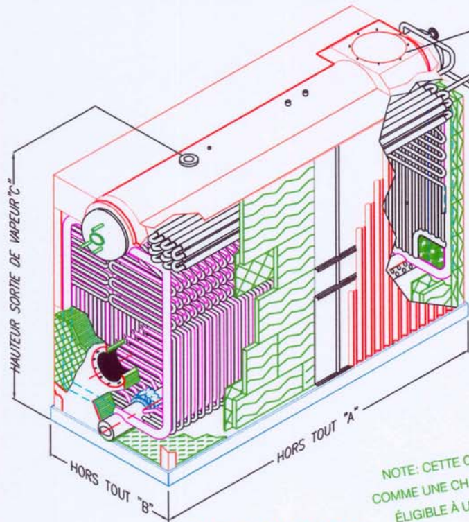
VUE AVANT DROITE
