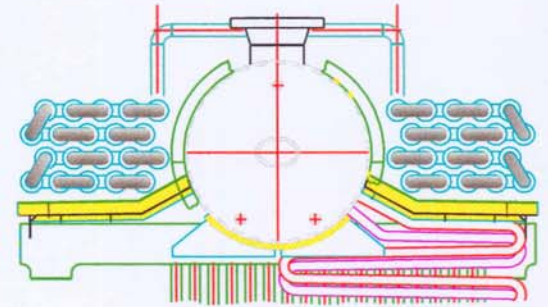
VUE AVANT ECONOMISEUR
